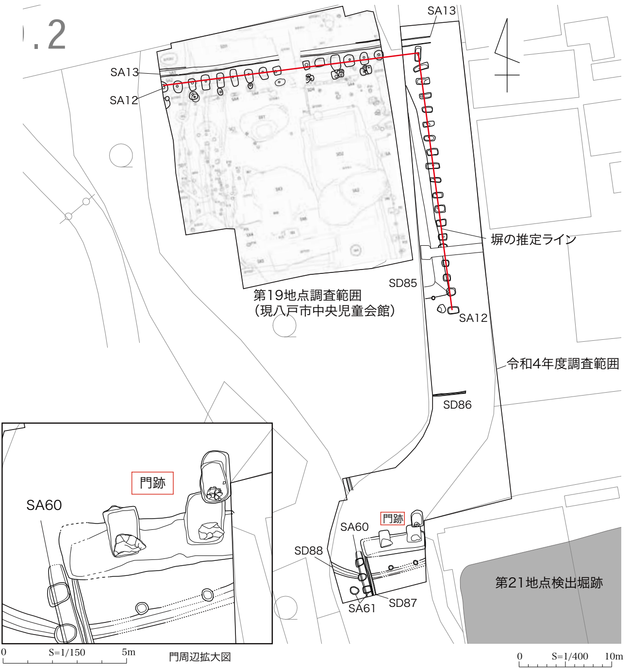
遺構配置図 八戸城跡第 54 地点
