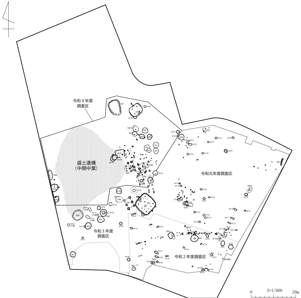
遺構配置図 松ヶ崎遺跡第 11 地点
